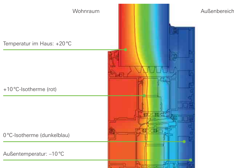
Querschnitt einer hochwärmegegedämmten Aluminium Haustür von Schüco. Der Isothermenverlauf zeigt: Trotz der Minusgrade außen herrscht auch direkt an der Haustür eine angenehme Innentemperatur
